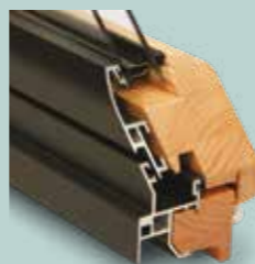
Double joint à frappe
