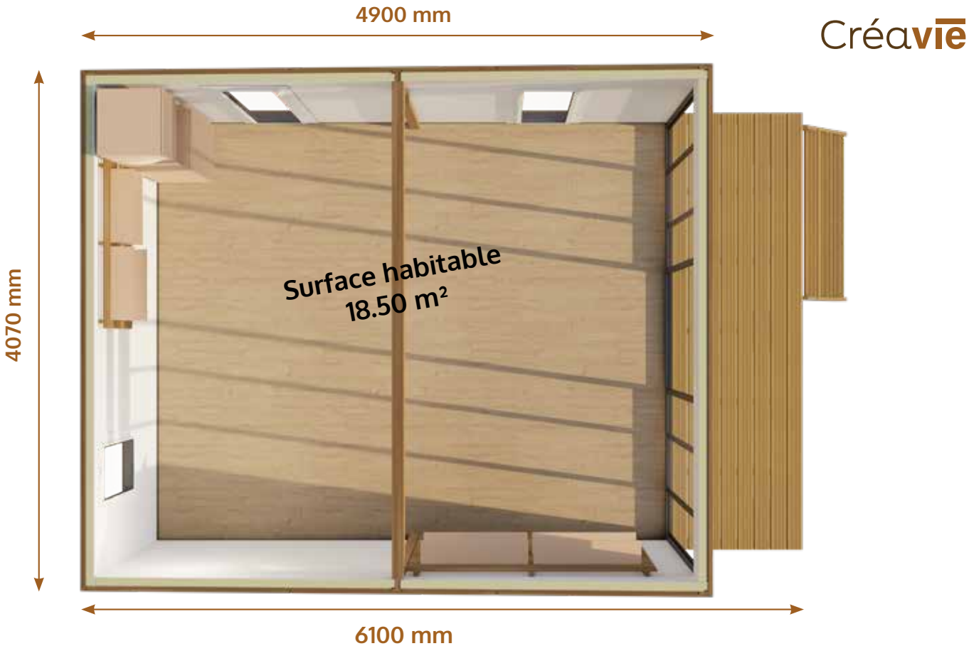
Dimensions exterieures
